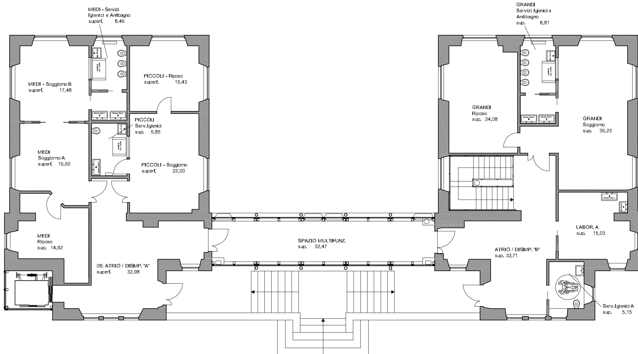
PIANO RIALZATO scala 1:100
