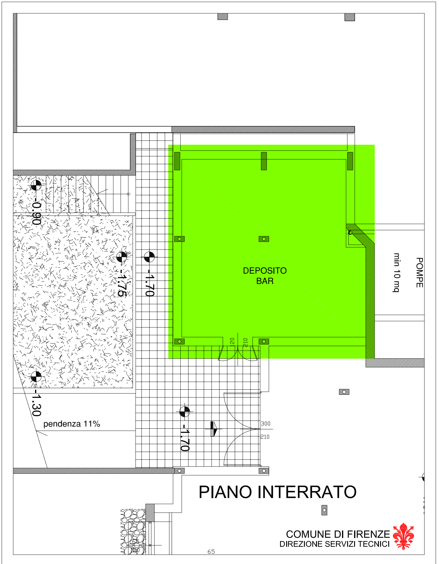
NUOVO CENTRO CULTURALE DI VIA CANOVA - FIRENZE PADIGLIONE 1 - BIBLIOTECA CANOVA Caffetteria - planimetria dei locali deposito (colore verde)
