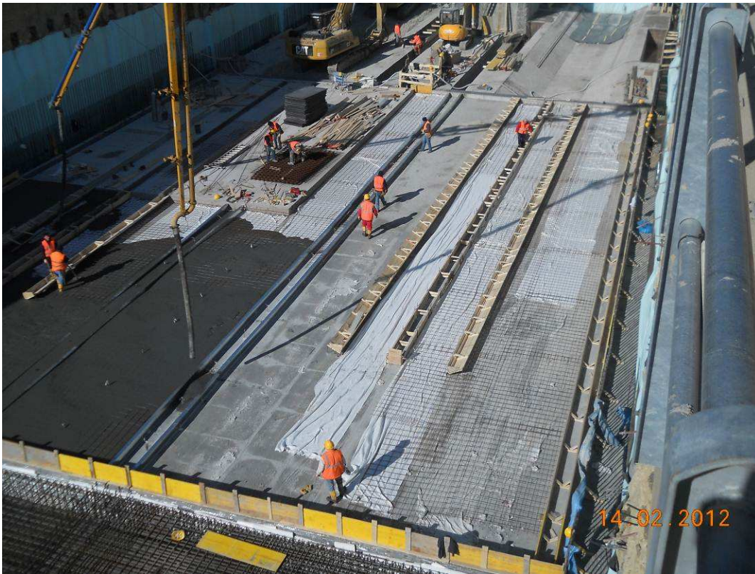
FOTO 1 – Pozzo Lancio Frese – getto di riempimento a protezione della soletta di fondazione
